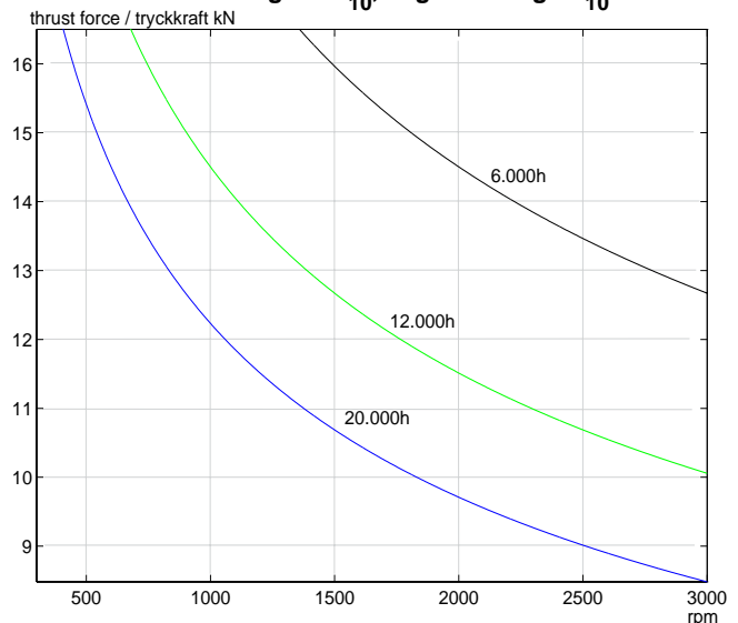
Bearing life L_{10} , Lagerlivslängd L_{10}
